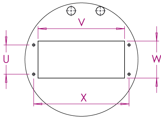
DETALLE A
